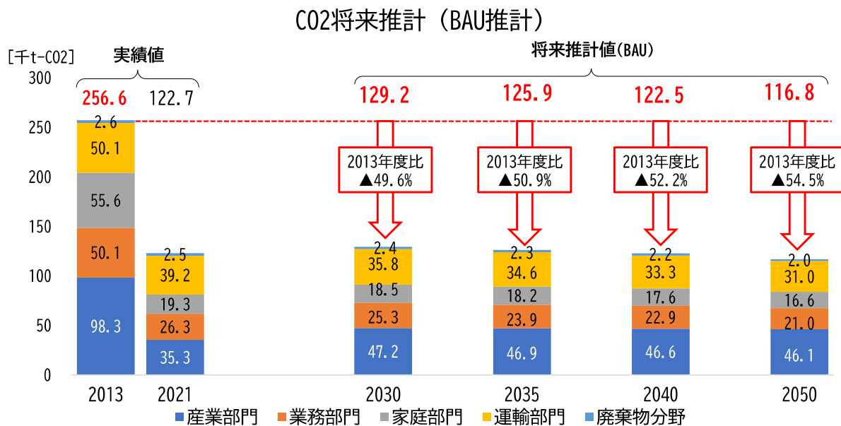
図 4-2-2 BAU 推計による将来 CO 2 排出量の推移
