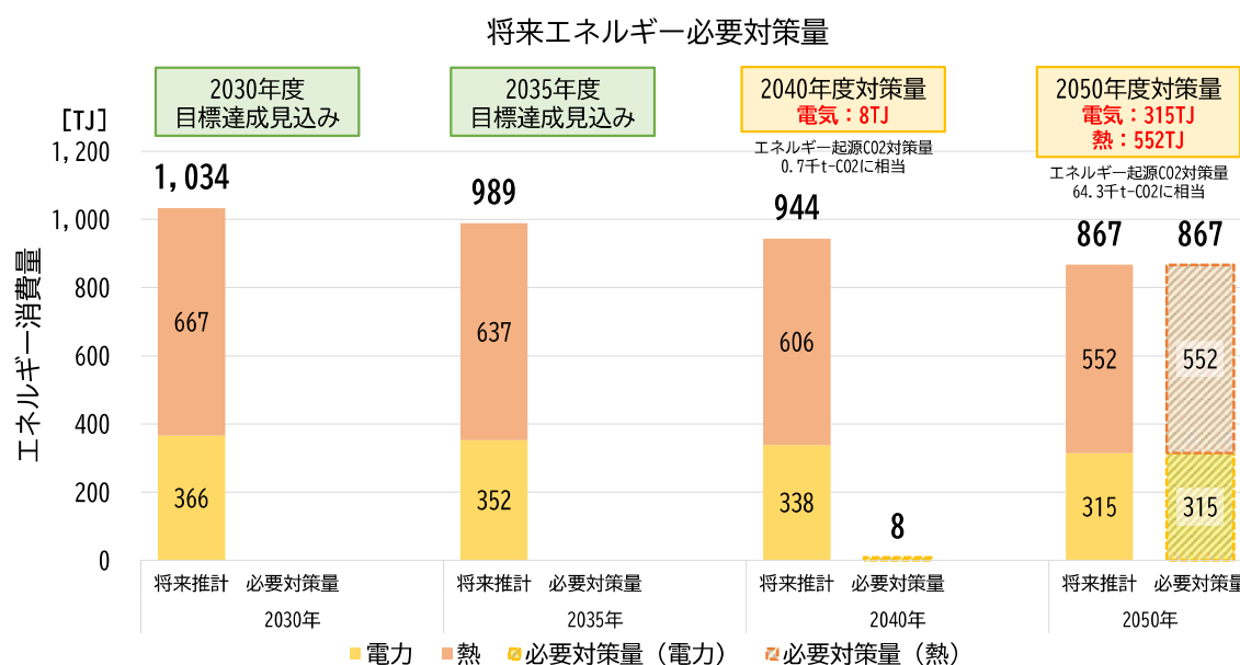
図 4-3-3 将来におけるエネルギー消費必要対策量
