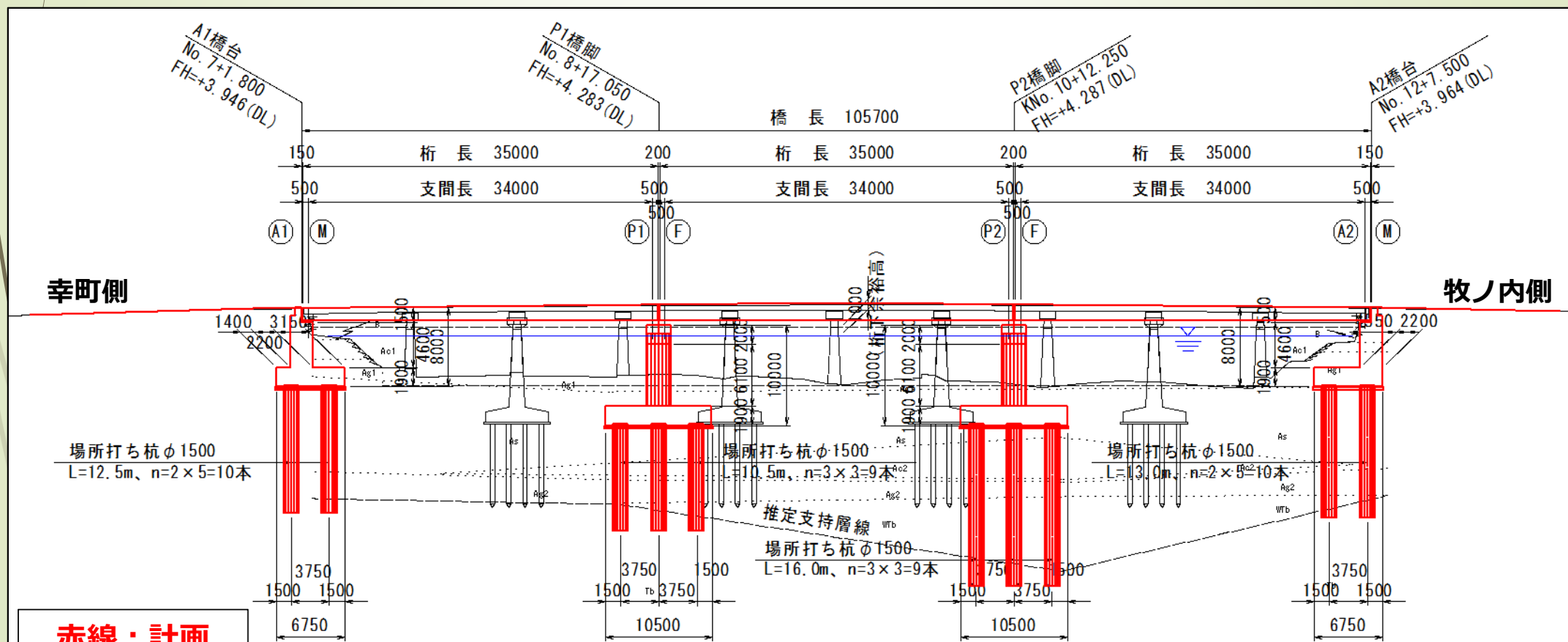
【 計画側面図 】
