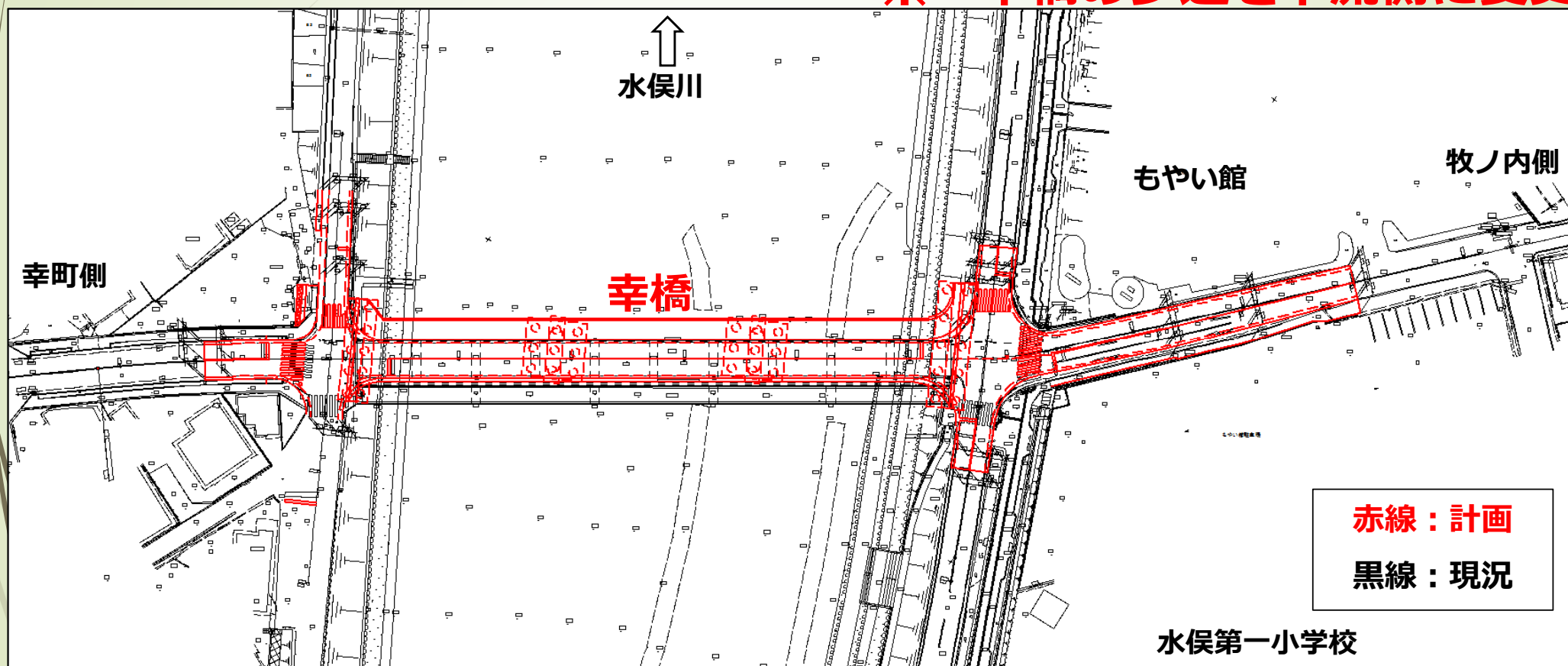
【 計画平面図 】
