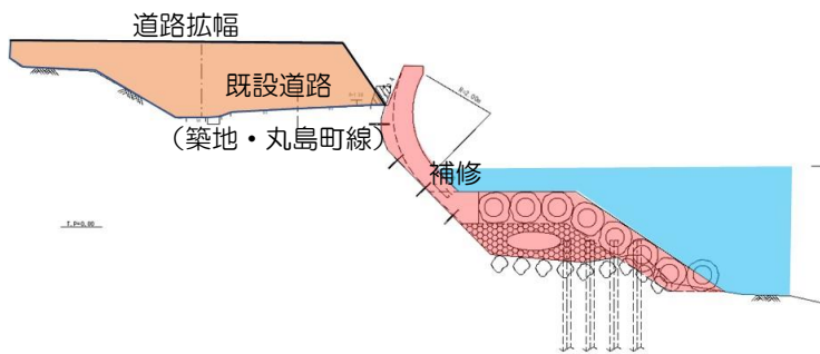
河口部断面イメージ
