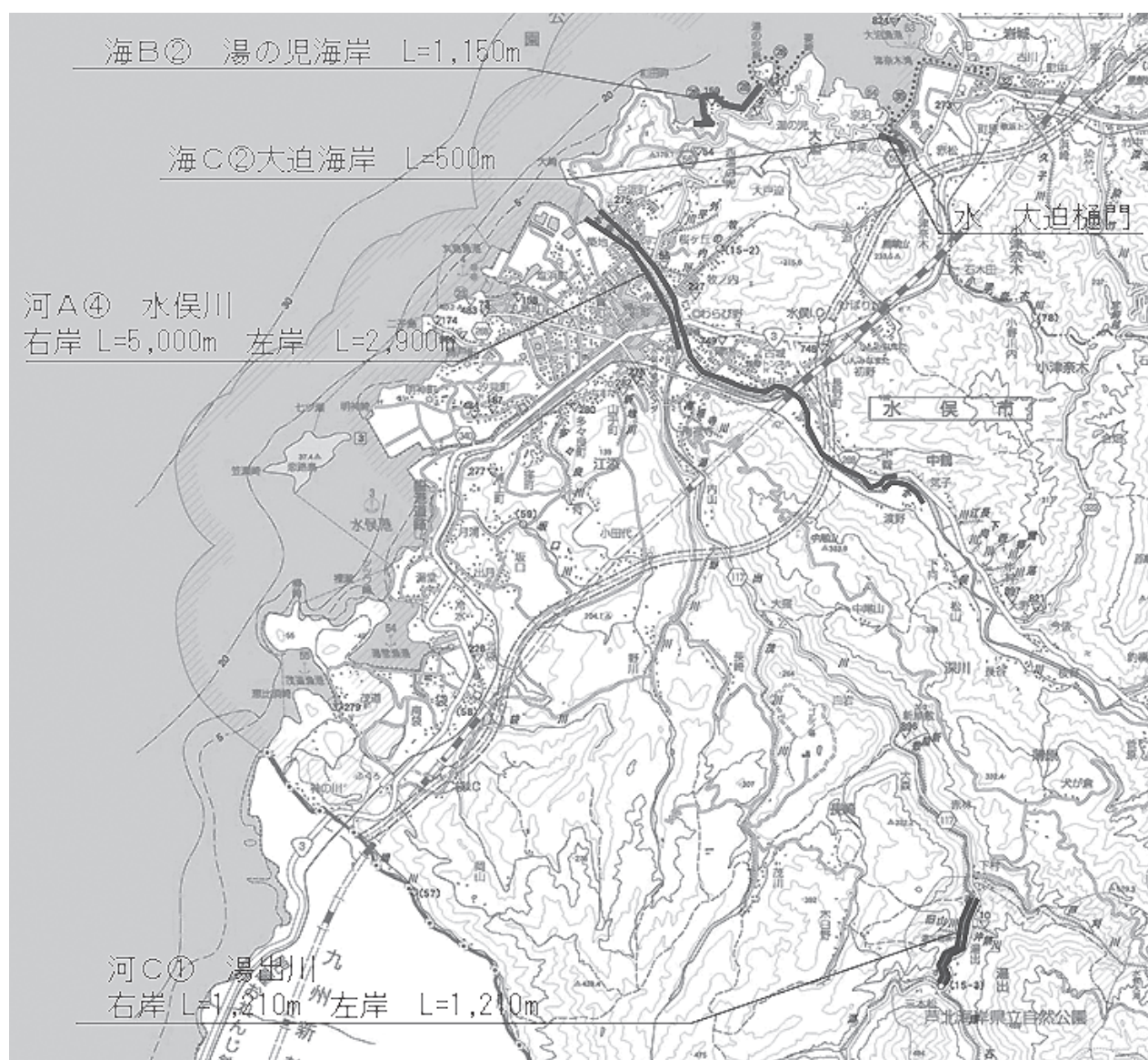
別図 重要水防区域図
